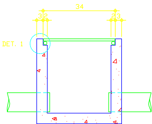
PLANTA ESCALA 1:10
