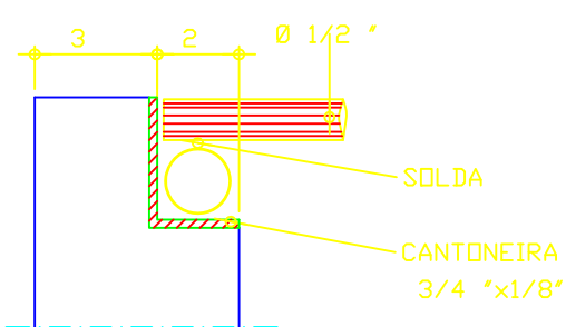
SEÇÃO 1-1 ESCALA 1:10
