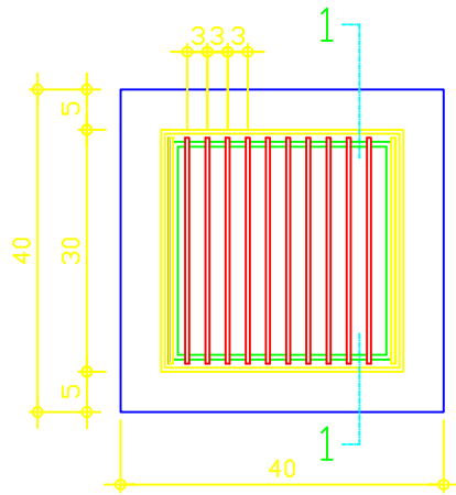
PLANTA ESCALA 1:10
